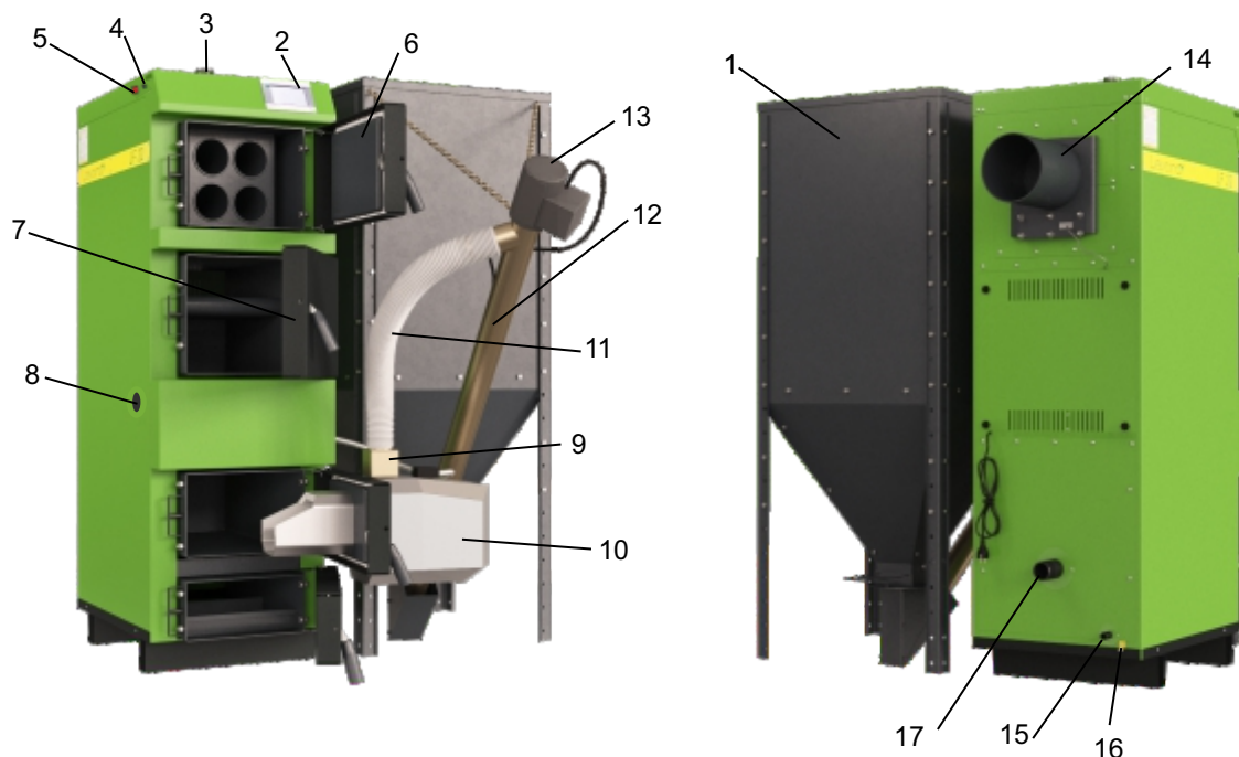
Рисунок 1. Состав и устройство Котлов моделей LF16-42
