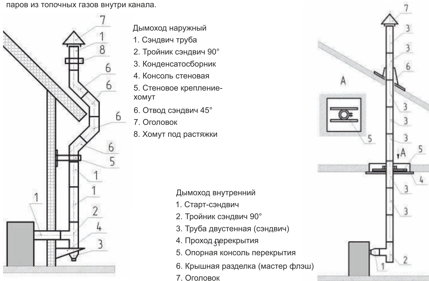
Рисунок Б.1. Пример сборки утепленного (сэндвич) дымохода по конденсату внутри и снаружи помещения
