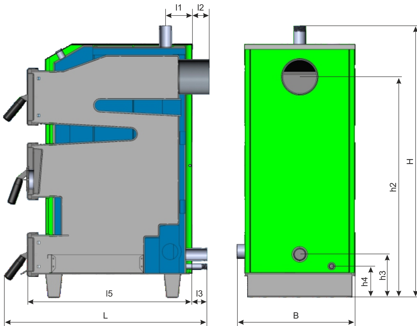
Рисунок 1. Габаритные и присоединительные размеры Котлов LAVORO есо серии «М» 10÷30 базовой комплектации.
