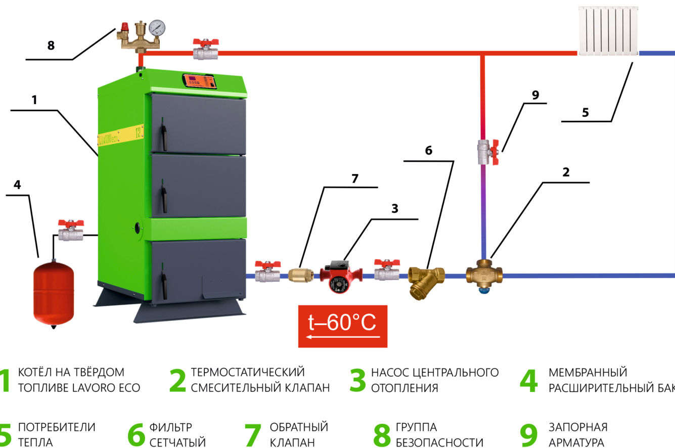
Рисунок 3. Типовая схема обвязки котла Lavoro Eco с 3-х ходовым клапаном
